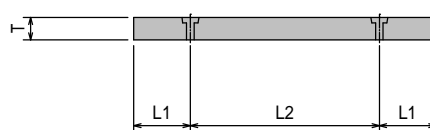
打ち込みボルト詳細図
