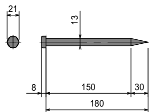
打ち込みボルト詳細図
